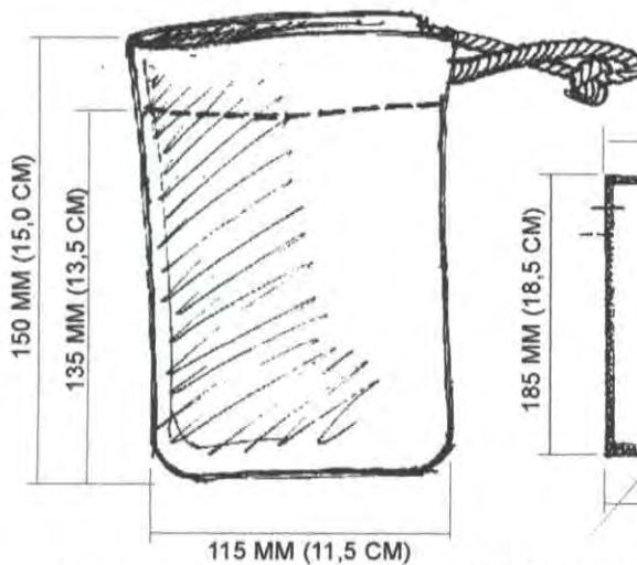
DIMENSIONES FINALES BOLSA TERMINADA
