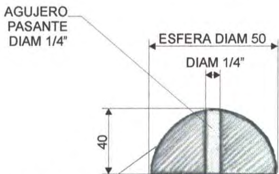
SECCIÓN A-A
