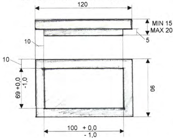
TAPA CONTENEDOR RECTÁNGULO
