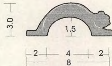
VISTA LATERAL
