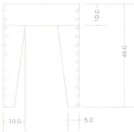
Pata en forma de ele Ensamble acolillado y con Tarugo
