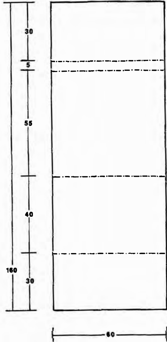
EJES PARA EJECUTAR LOS DOBLECES ESCALA 1 : 12,5
