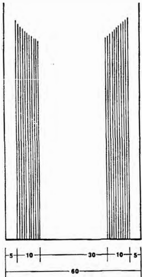
DISPOSICIÓN DE LAS FRANJAS EN EL URDIDO ESCALA 1 : 10
