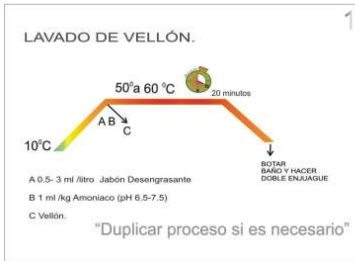
CURVA LAVADO DE VELLÓN
