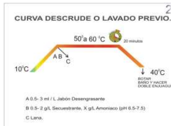
CURVA DE DESCRUDE Fuente: Carol Valencia C. 2007
