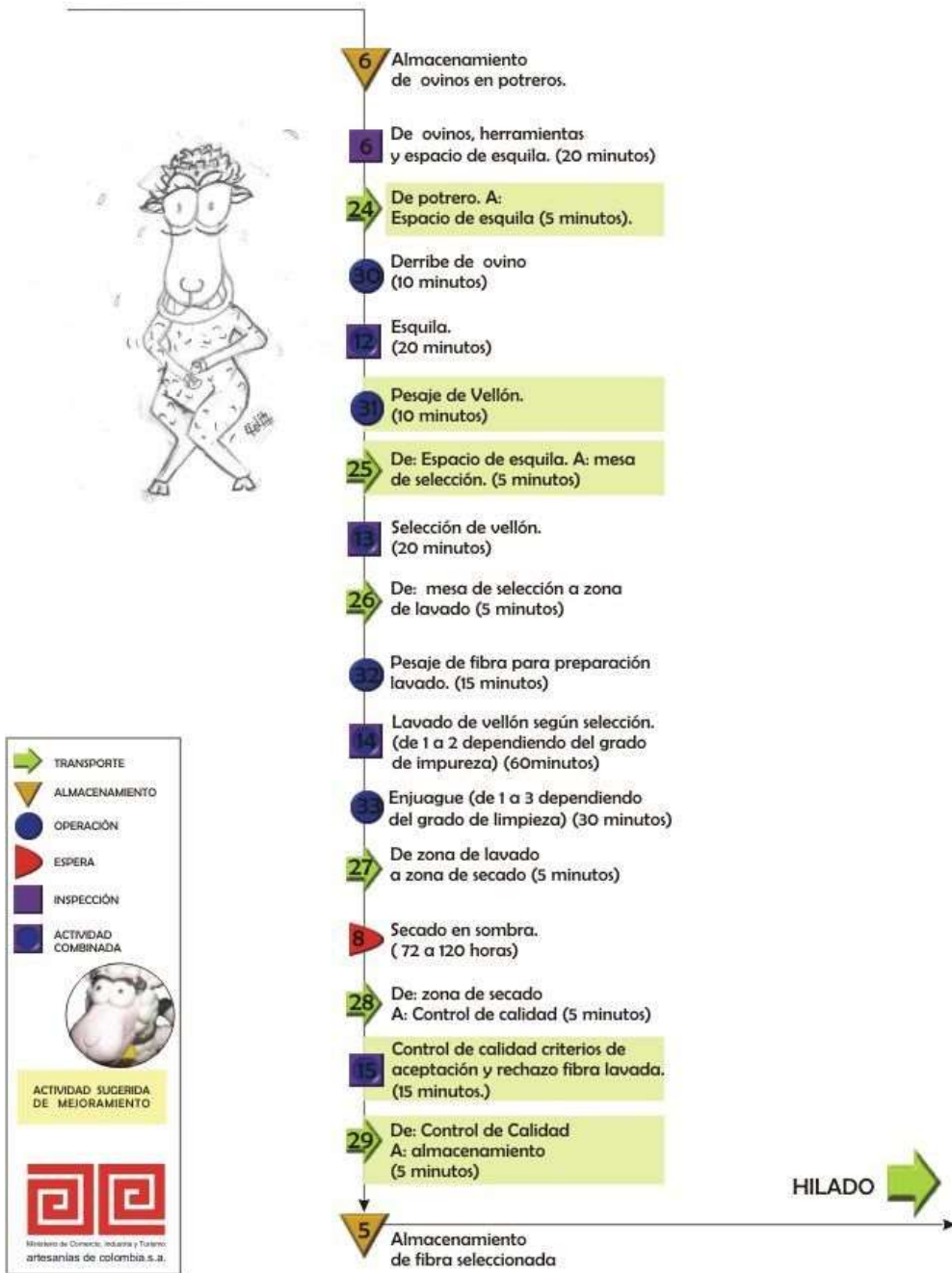
DIAGRAMA DE FLUJO ESQUILA, PROPUESTA Fuente: Carol Valencia C.2007
