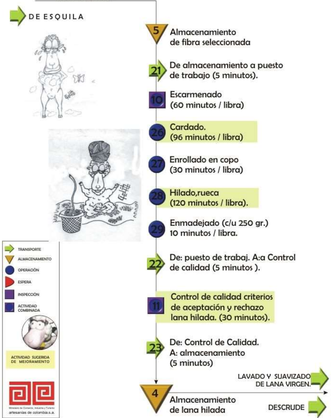
DIAGRAMA DE FLUJO HILADO, PROPUESTA Fuente: Carol Valencia C.2007
