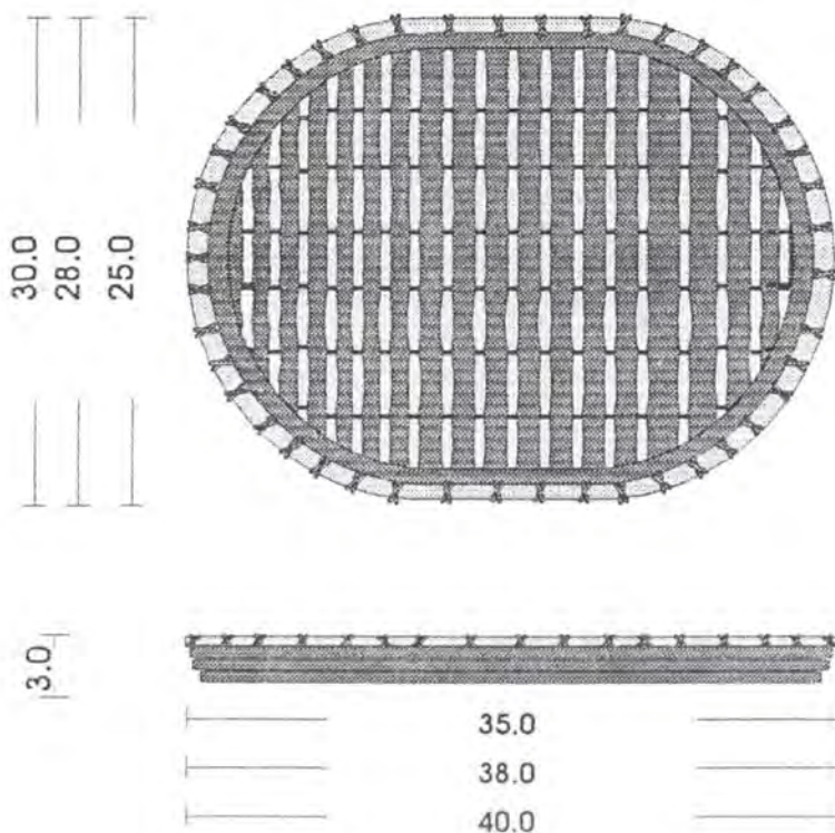
VISTA SUPERIOR
